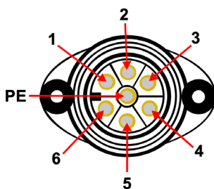
Belegung Buchsen-/Steckerteil
